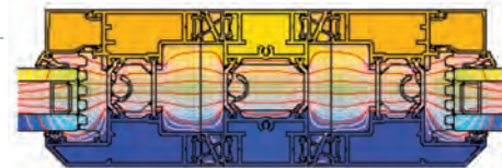
przekrój przez skrzydło (skrzydło typ A) – Panorama i+
