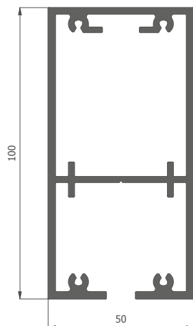
NF001 profilé du guidage
