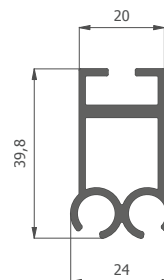
NF200 profilé de la poutre anti-vent
